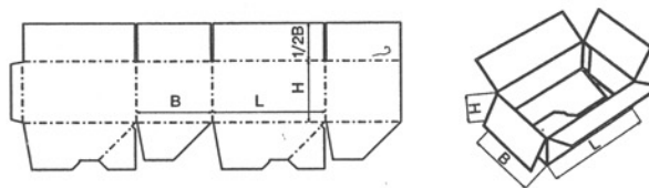
FEFCO 0712
