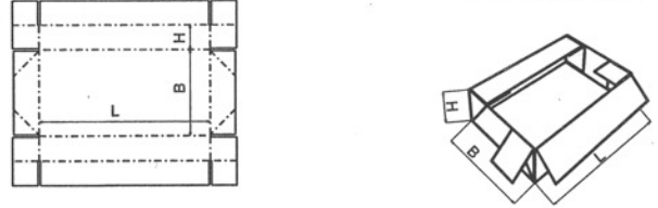
FEFCO 0747
