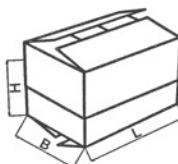
FEFCO 0321
