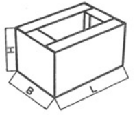
FEFCO 0210
