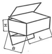
FEFCO 0204
