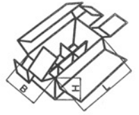
FEFCO 0209
