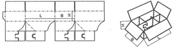
FEFCO 0718
