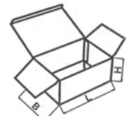
FEFCO 0216
