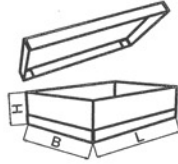
FEFCO 0311
